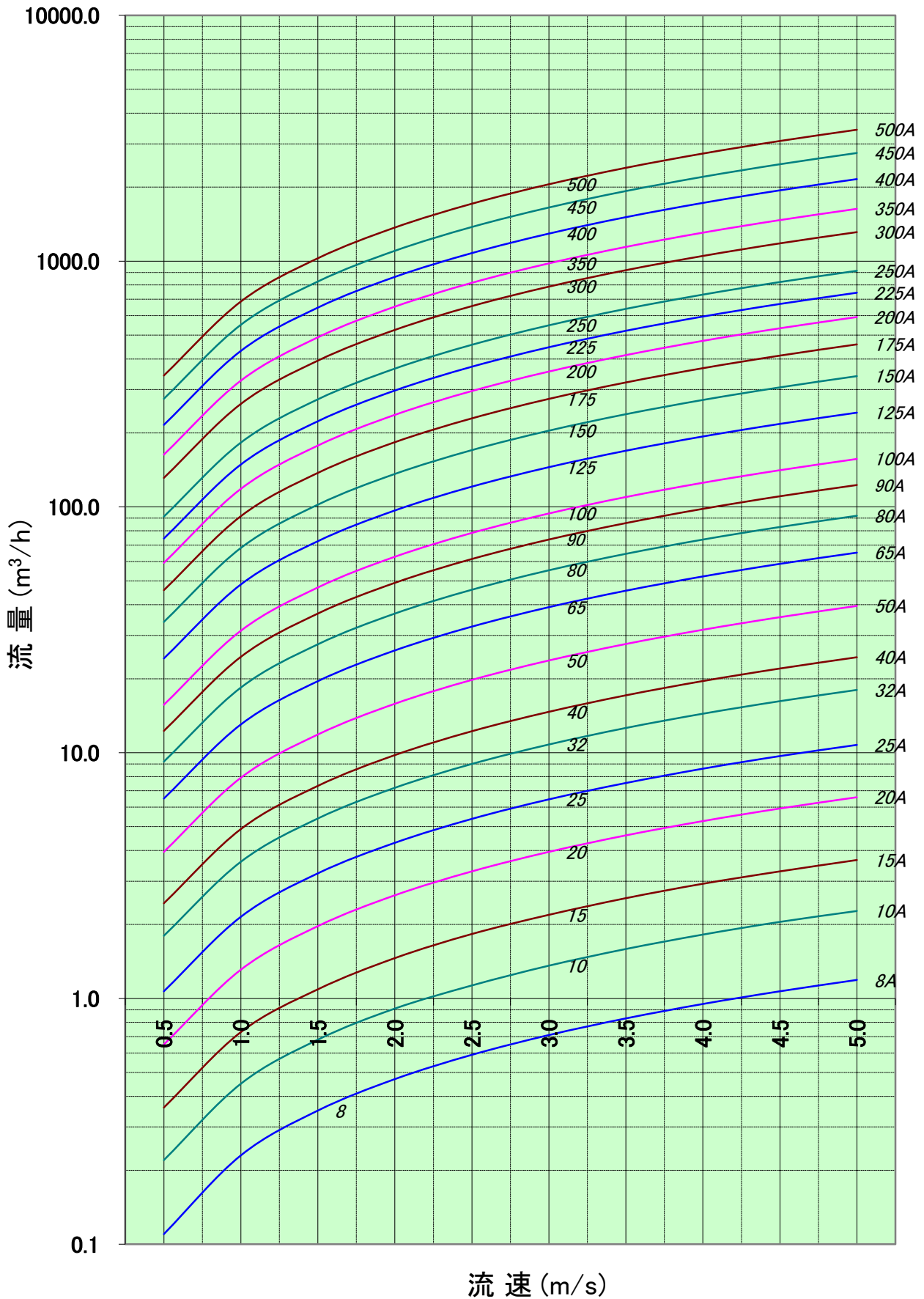
各配管サイズと流速の流量曲線
